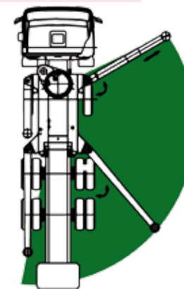
ST-talpalás ST-Abstützung
